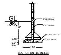
SECTION ON - BB (N.T.S)
