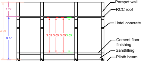
SECTION - AB
