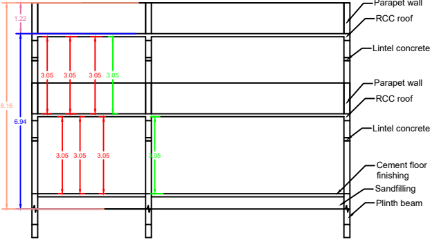
SECTION - AB
