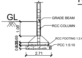
SECTION ON - BB (N.T.S)
