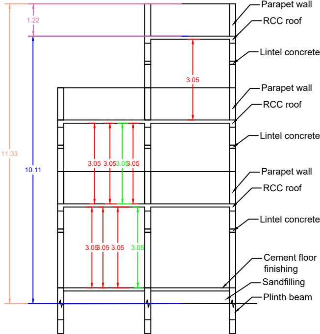
SECTION - AB
