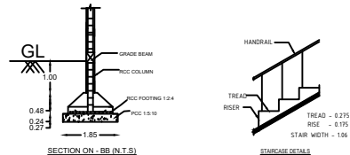
SECTION ON - BB (N.T.S.)
