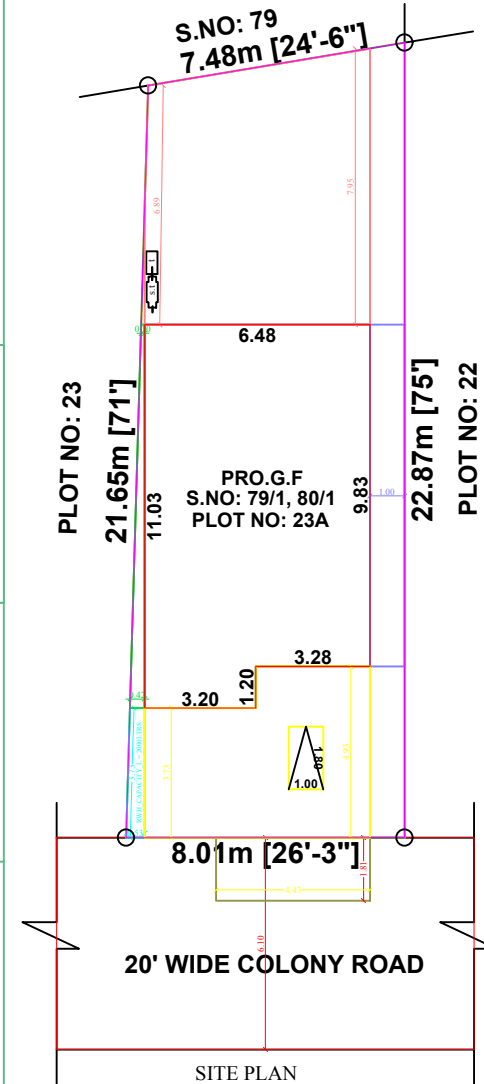
SITE PLAN SCALE 1:100
