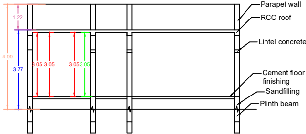
SECTION - AB
