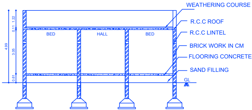
SECTION - AB
