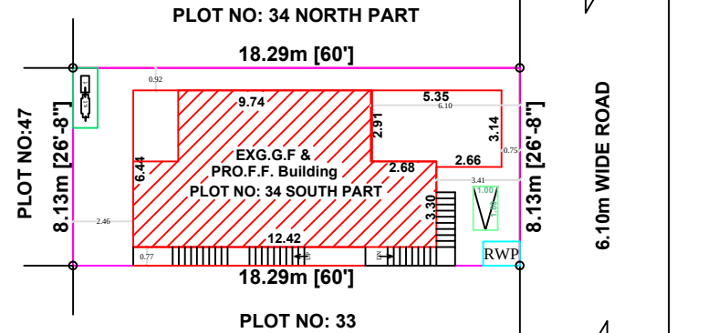
SITE PLAN SCALE 1:100
