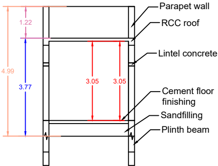
SECTION - AB
