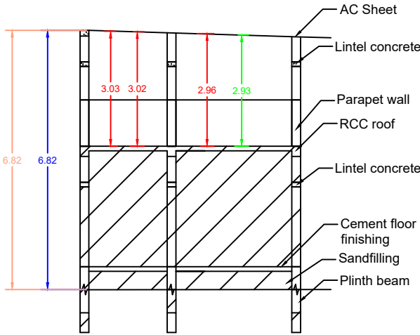
SECTION - AB
