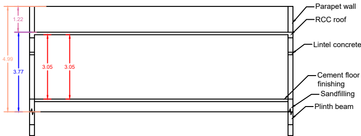
SECTION - AB
