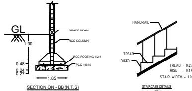
SECTION ON - BB (N.T.S)
