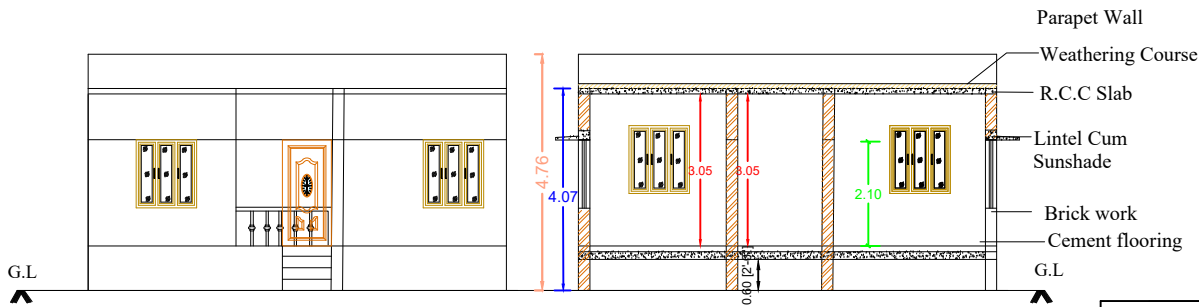
ELEVATION
