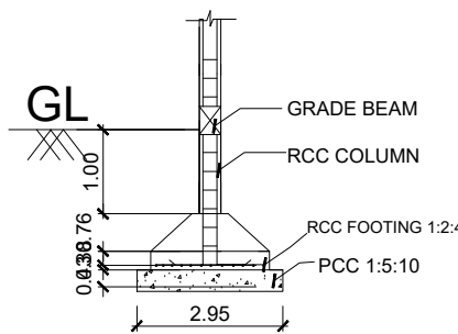
SECTION ON - BB (N.T.S)
