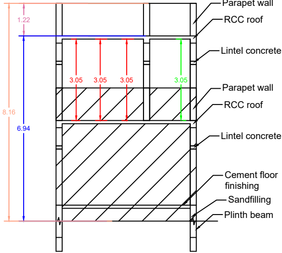
SECTION - AB
