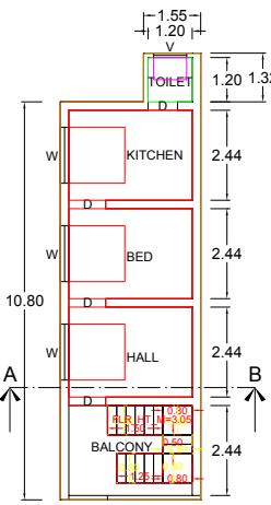
F.F. PLAN
