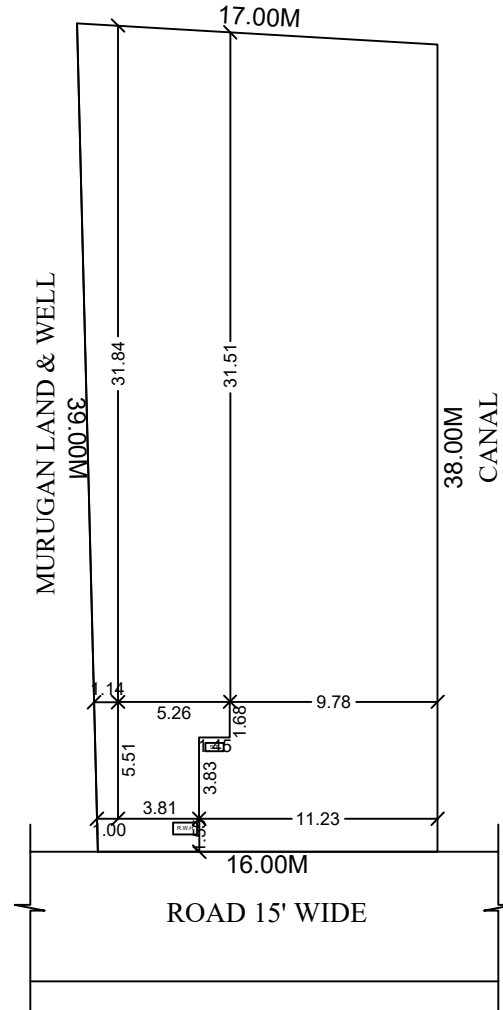
SITE PLAN (1:300)
