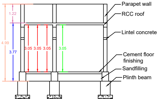
SECTION - AB
