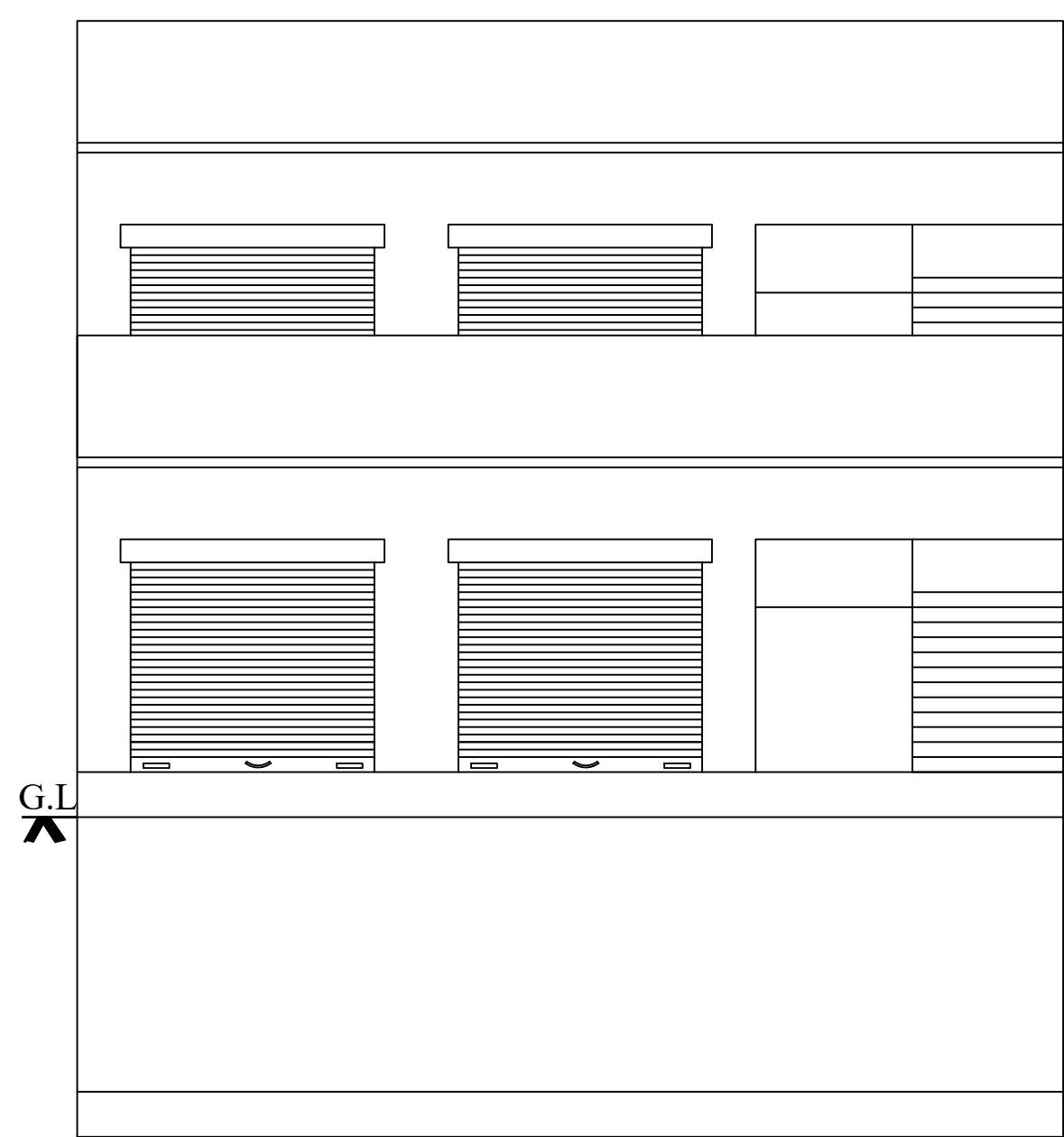
ELEVATION
