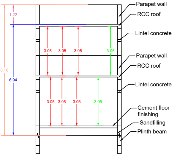
SECTION - AB
