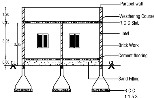
SECTION ON'AB'
