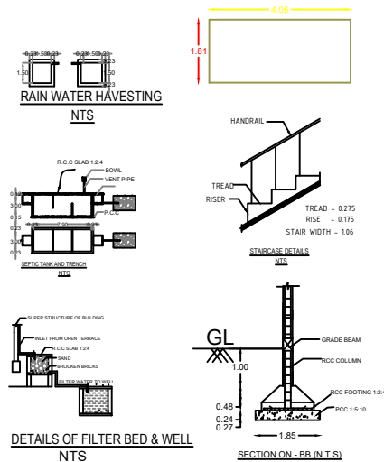
SECTION ON - BB (N.T.S.)
