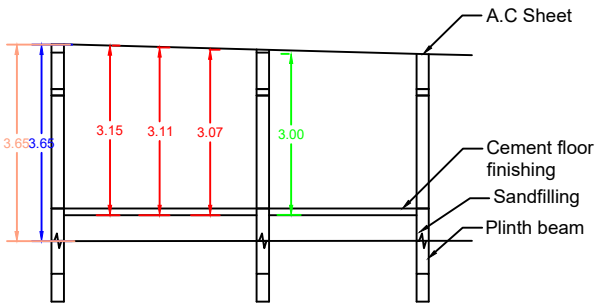
SECTION - AB
