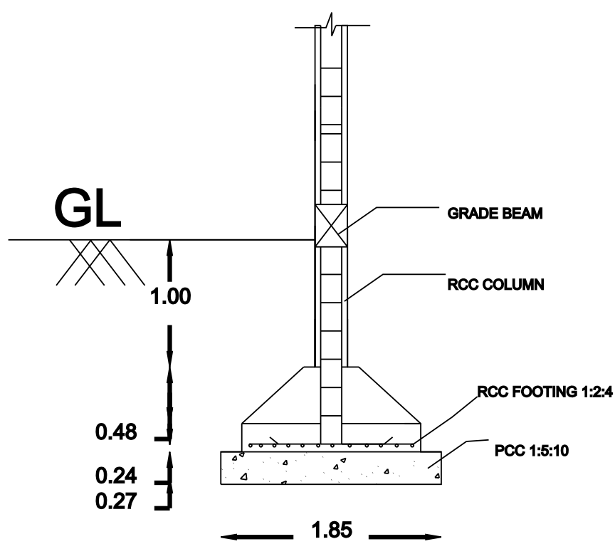
SECTION ON - BB (N.T.S)
