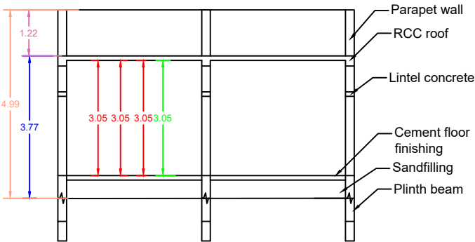
SECTION - AB
