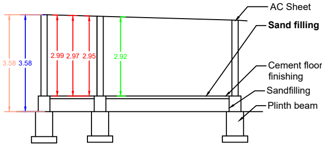
SECTION - AB
