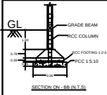
SECTION ON - BB (N.T.S)
