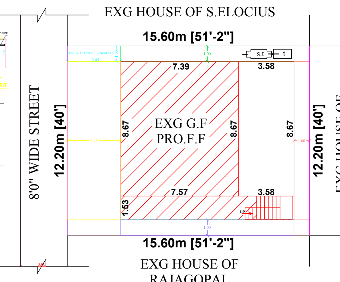
SITE PLAN 1:100
