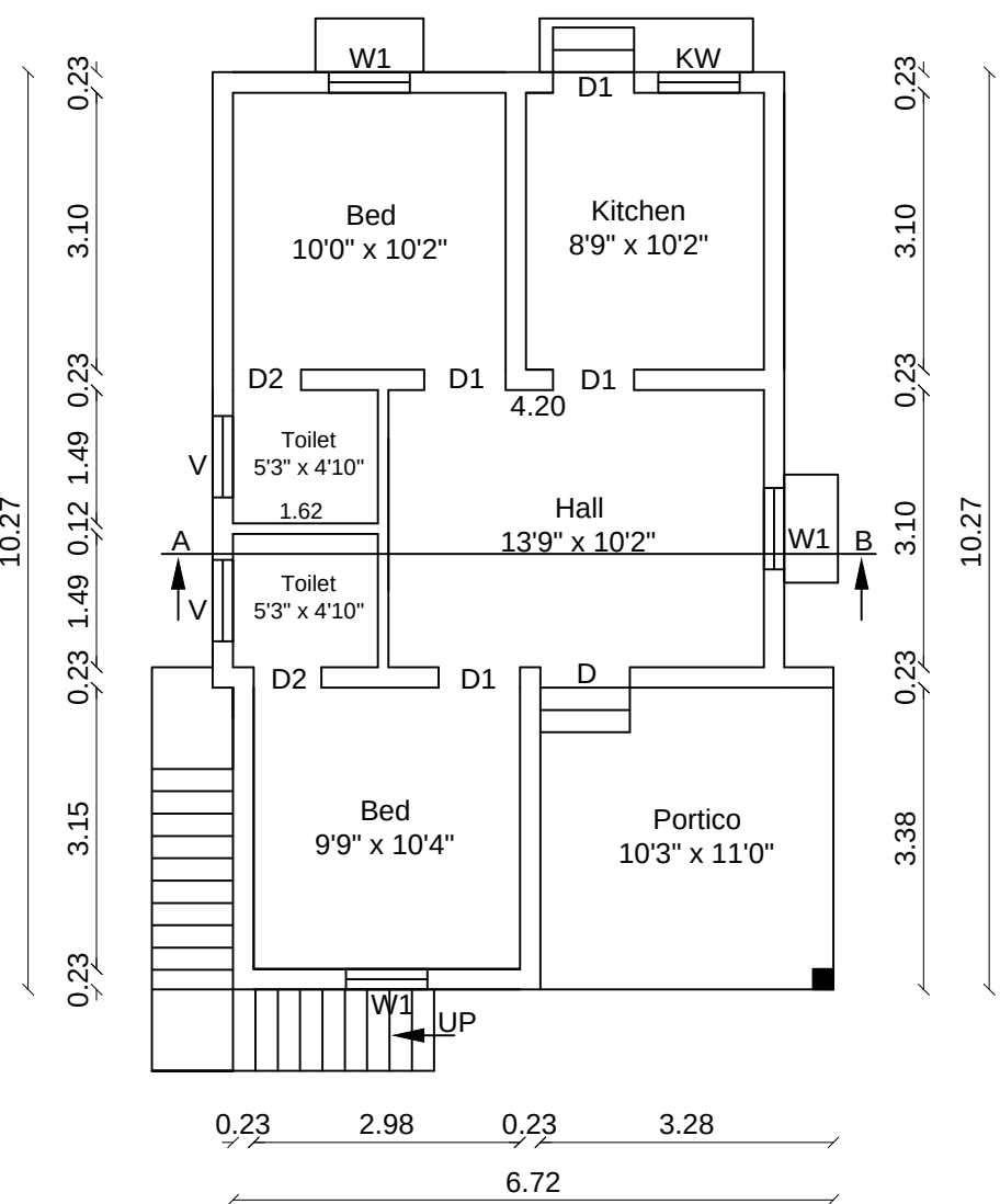
EXG G.F PLAN
