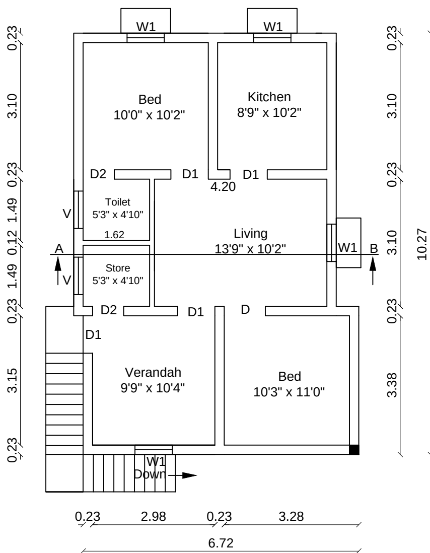
PRO F.F PLAN
