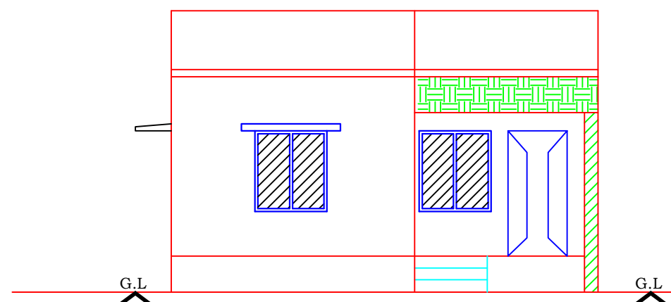
ELEVATION
