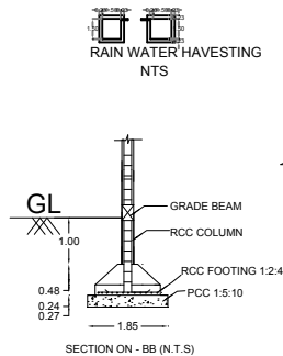
SECTION ON - BB (N.T.S)
