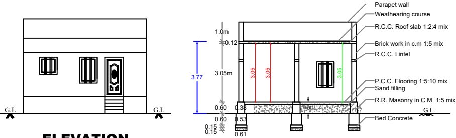
ELEVATION
