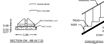
SECTION ON - BB (N.T.S)
