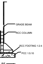
SECTION ON - BB (N.T.S)
