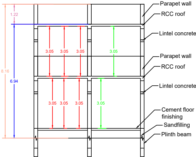
SECTION - AB
