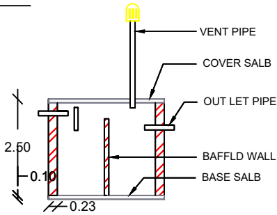
SECTION ON X - Y
