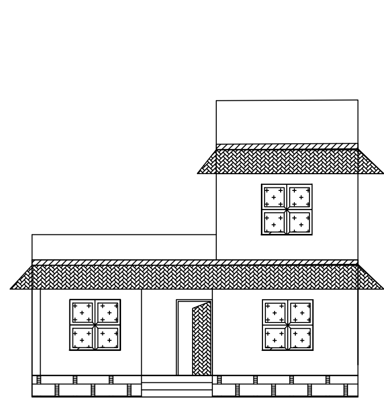
ELEVATION
