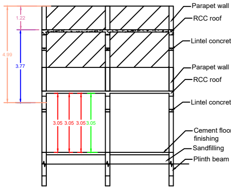
SECTION - AB
