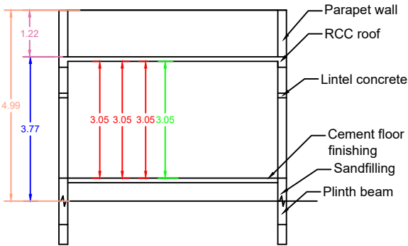
SECTION - AB
