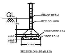
SECTION ON - BB (N.T.S)
