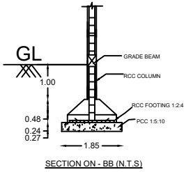
SECTION ON - BB (N.T.S)
