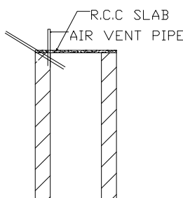
SOAK PIT
