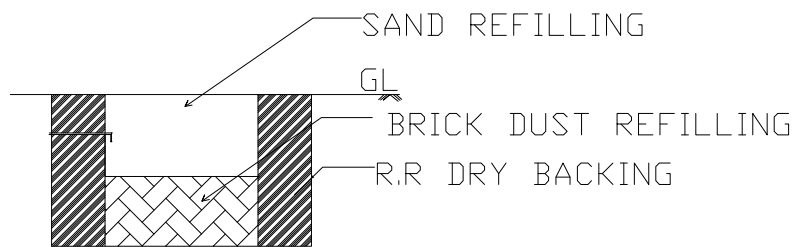
SOAK PIT
