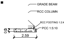
SECTION ON - BB (N.T.S)
