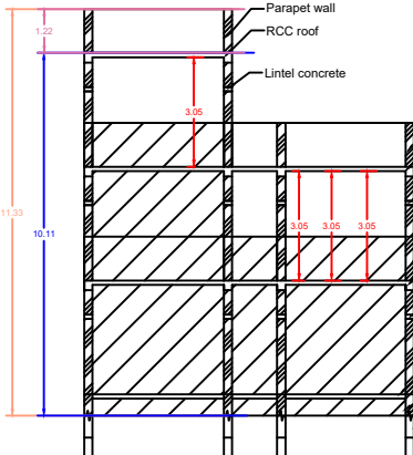
SECTION - AB
