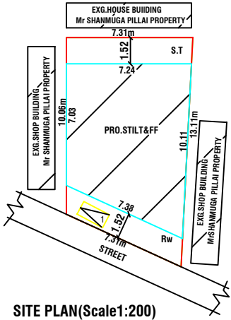
SITE PLAN(Scale1:200)
