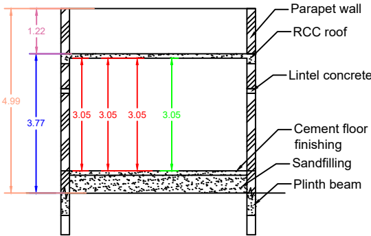
SECTION - AB
