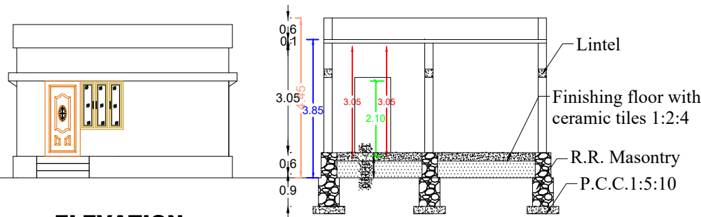
ELEVATION
