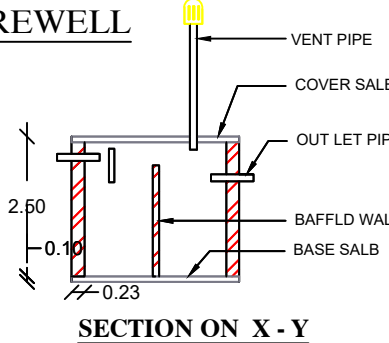
SECTION ON X - Y
